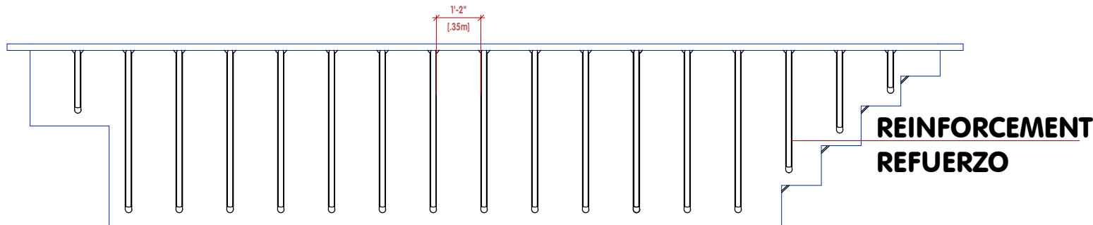
LONGITUDINAL SIDE VIEW C-C VISTA LATERAL LONGITUDINAL C-C
