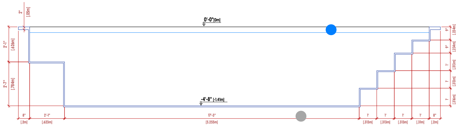
LONGITUDINAL SECTION A-A SECCIÓN LONGITUDINAL A-A
