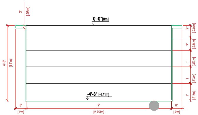
CROSS SECTION B-B SECCIÓN TRANSVERSAL B-B
